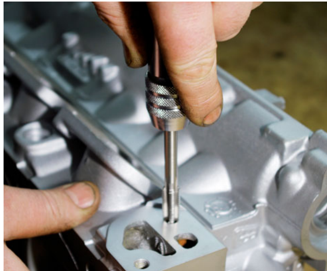
Schneiden des HELICOIL® Aufnahmegewindes mit dem kombinierten Bohr- und Schneidwerkzeug.
