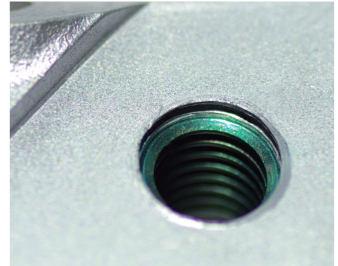
HELICOIL® Plus in eingebautem Zustand.
