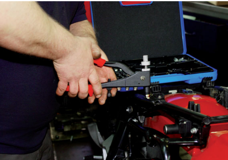
Setzen der RIVKLE® Blindnietmutter M6 in den Motorradrahmen.
