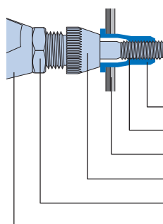
Ecrou RIVKLE®
