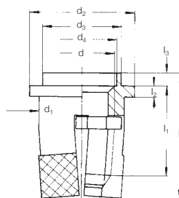
Typ 0232 EXPANSIONSSERT 1 Clinch
